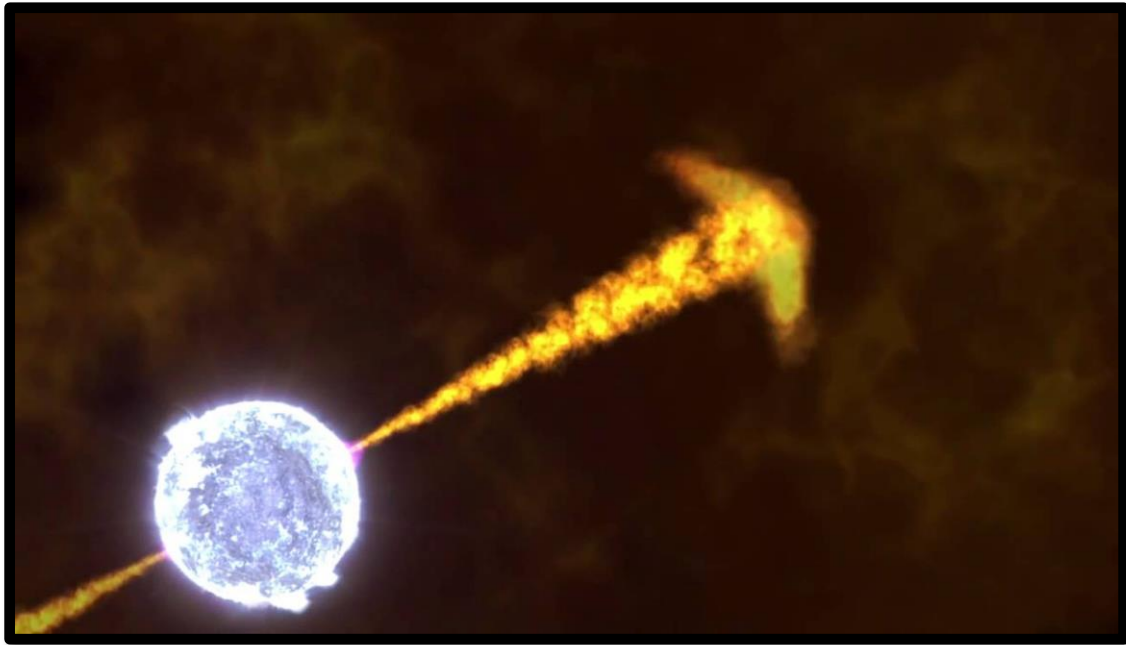
Video: Gammablitz 130427A
